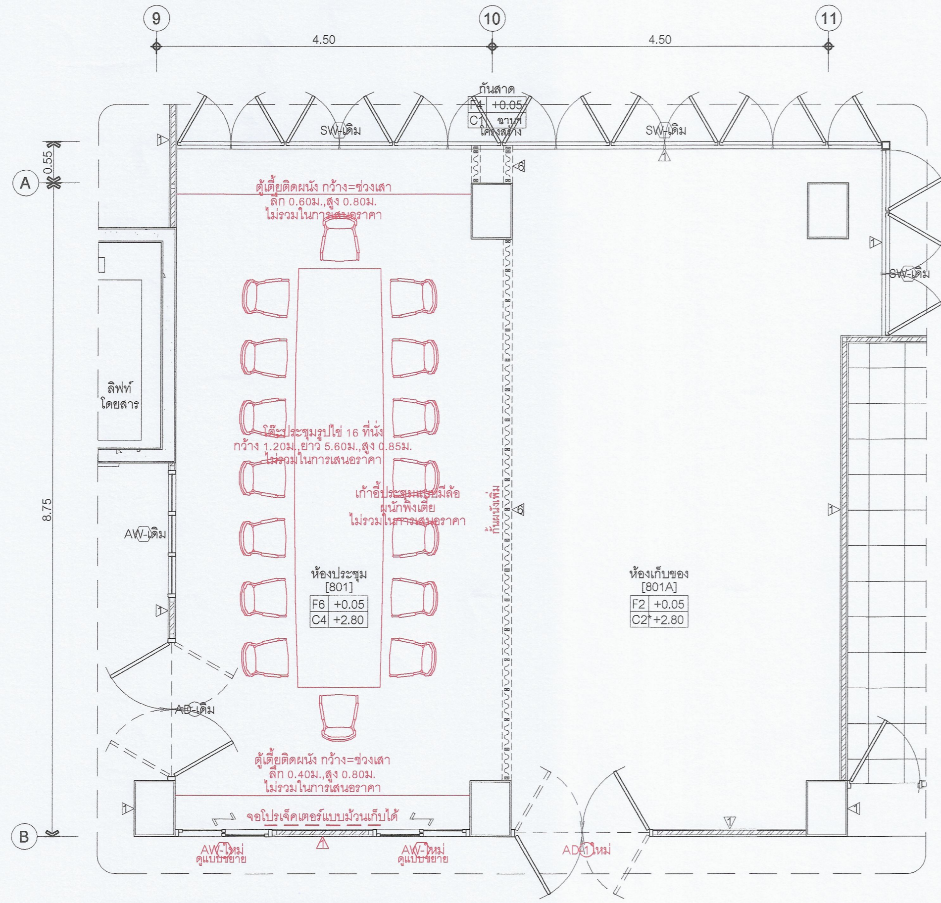
แปลนขยายห้องประชุม ชั้น 8 หลังปรับปรุง แสดงแปลนเพดานฝ้า 1:50
