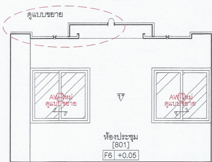
รูปด้าน [1] ห้องประชุม ชั้น 8 หลังปรับปรุง มาตราส่วน 1:50
