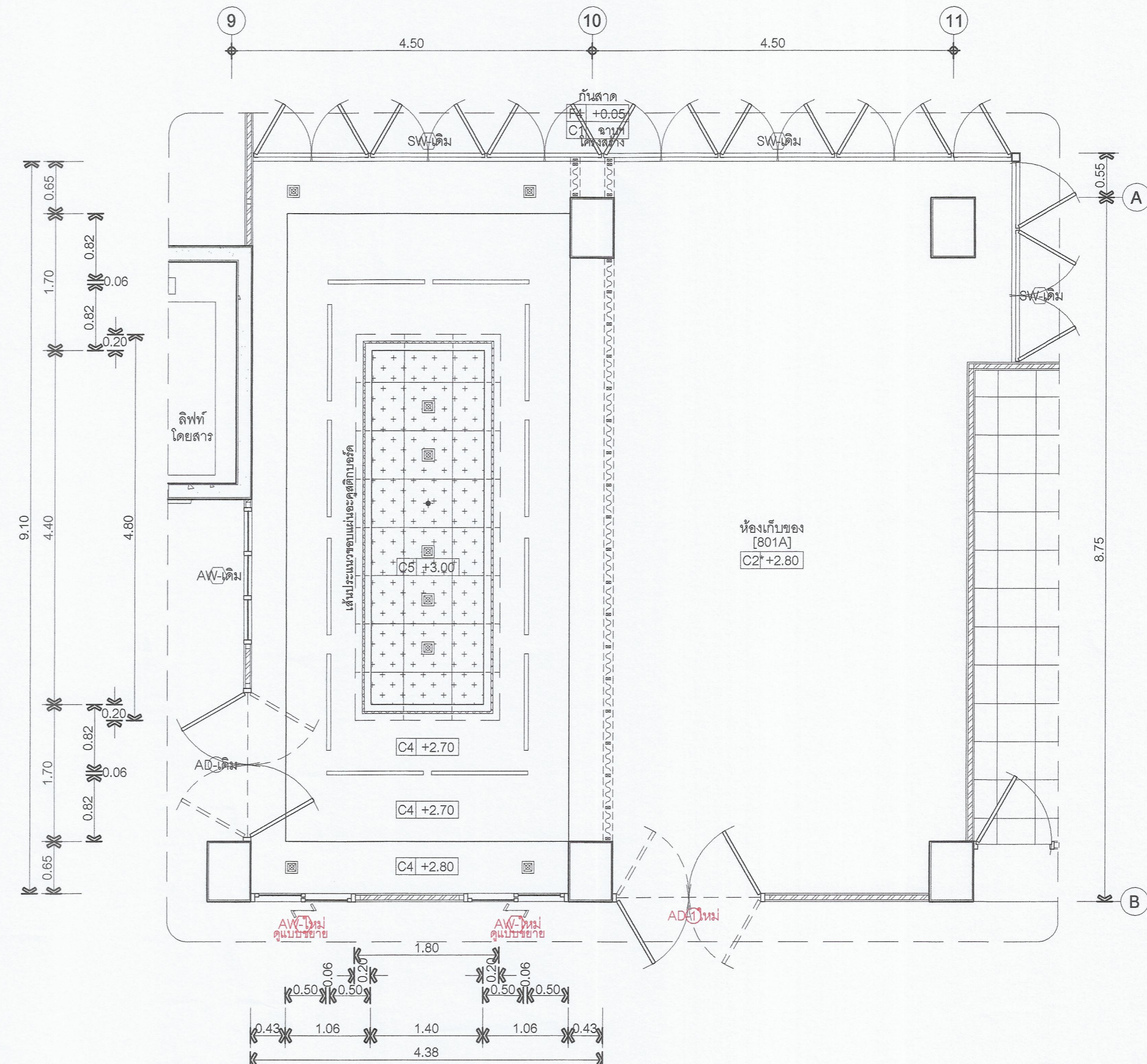
แปลนขยายห้องประชุม ชั้น 8 หลังปรับปรุง แสดงแปลนฝ้าเพดาน 1:50
