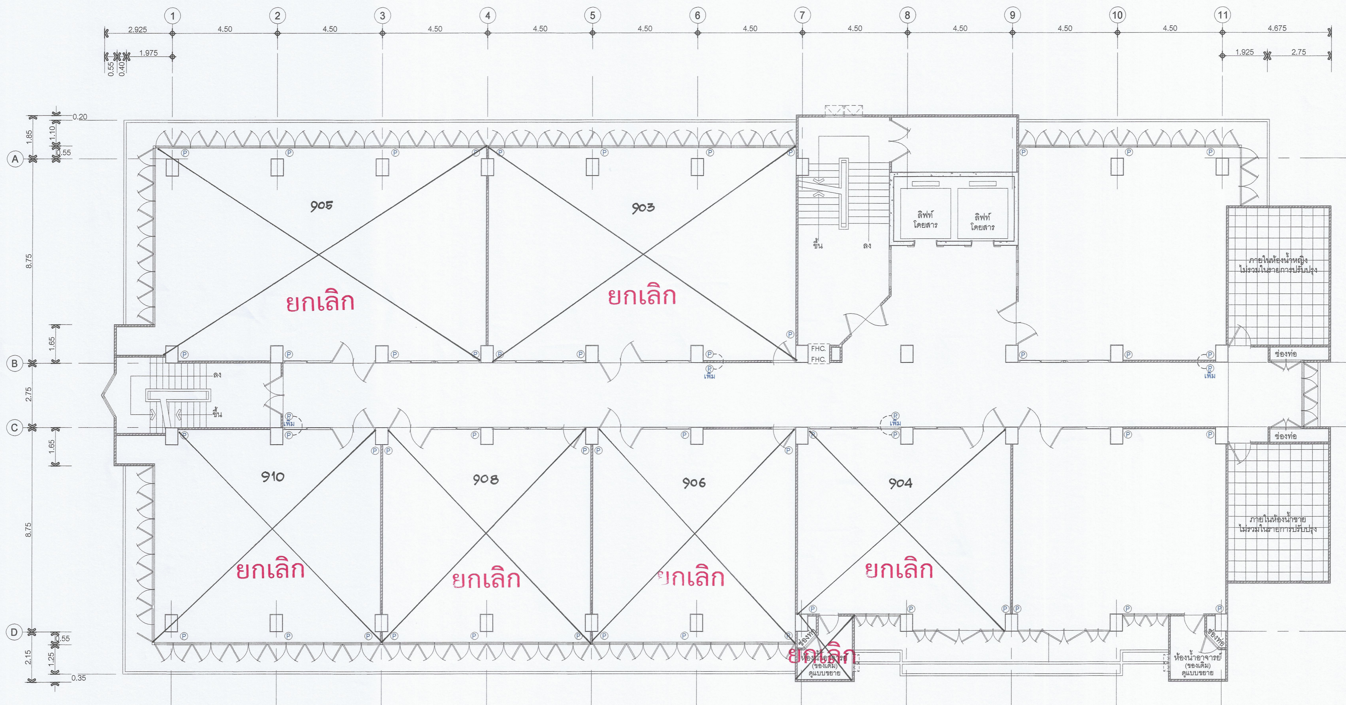
9th. FLOOR PLAN ไฟฟ้าเต้าเสียบ หลังปรับปรุง มาตราส่วน 1 : 100
