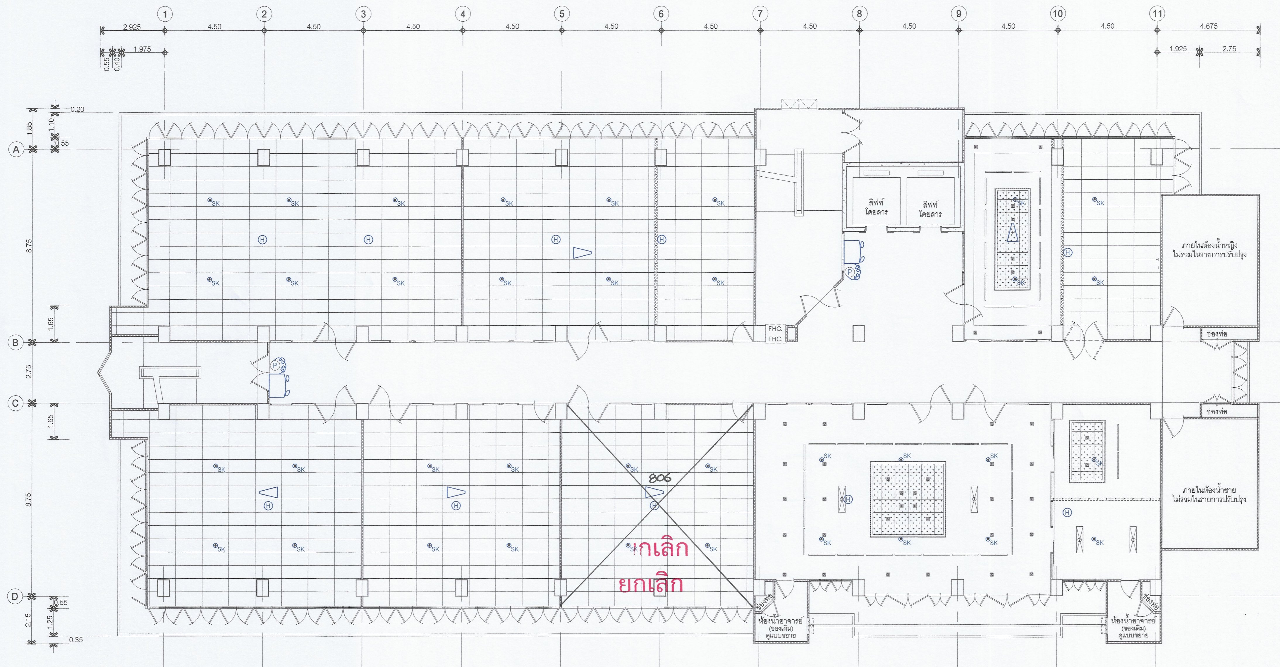
8th. FLOOR PLAN ไฟฉุกเฉิน,เครื่องPROJECTOR SPRINKLER,HEAT DETECTOR หลังปรับปรุง มาตราส่วน 1 : 100
