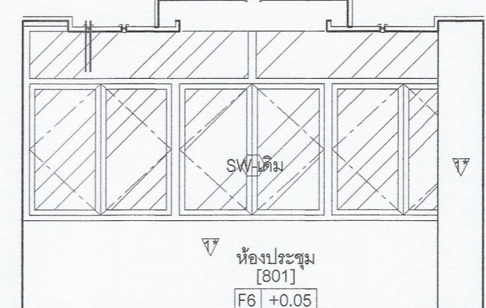
รูปด้าน [3] ห้องประชุม ชั้น 8 หลังปรับปรุง มาตราส่วน 1:50
