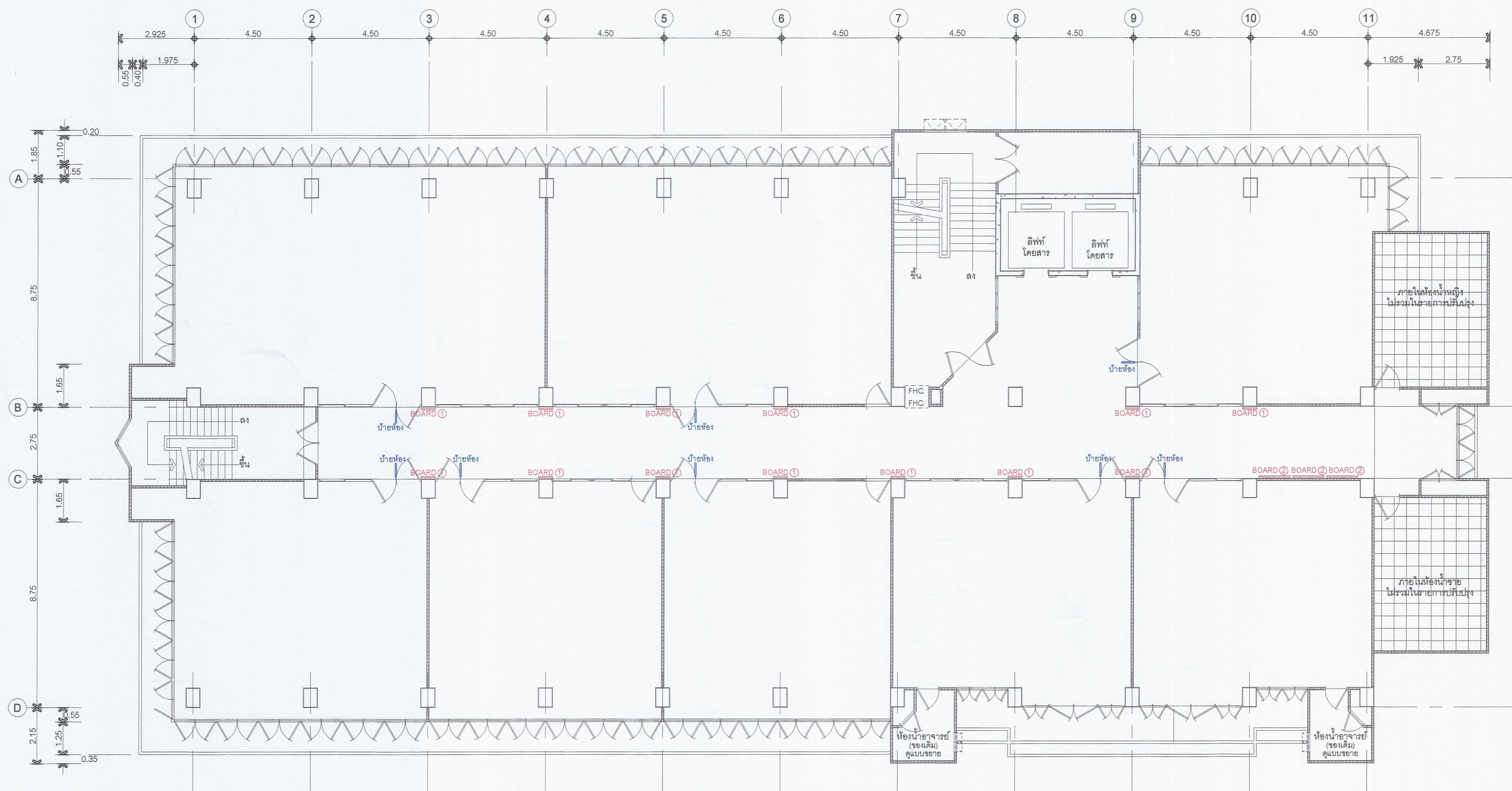
9th. FLOOR PLAN แสดงอุปกรณ์ประกอบในแต่ละชั้น หลังปรับปรุง มาตราส่วน 1:100
