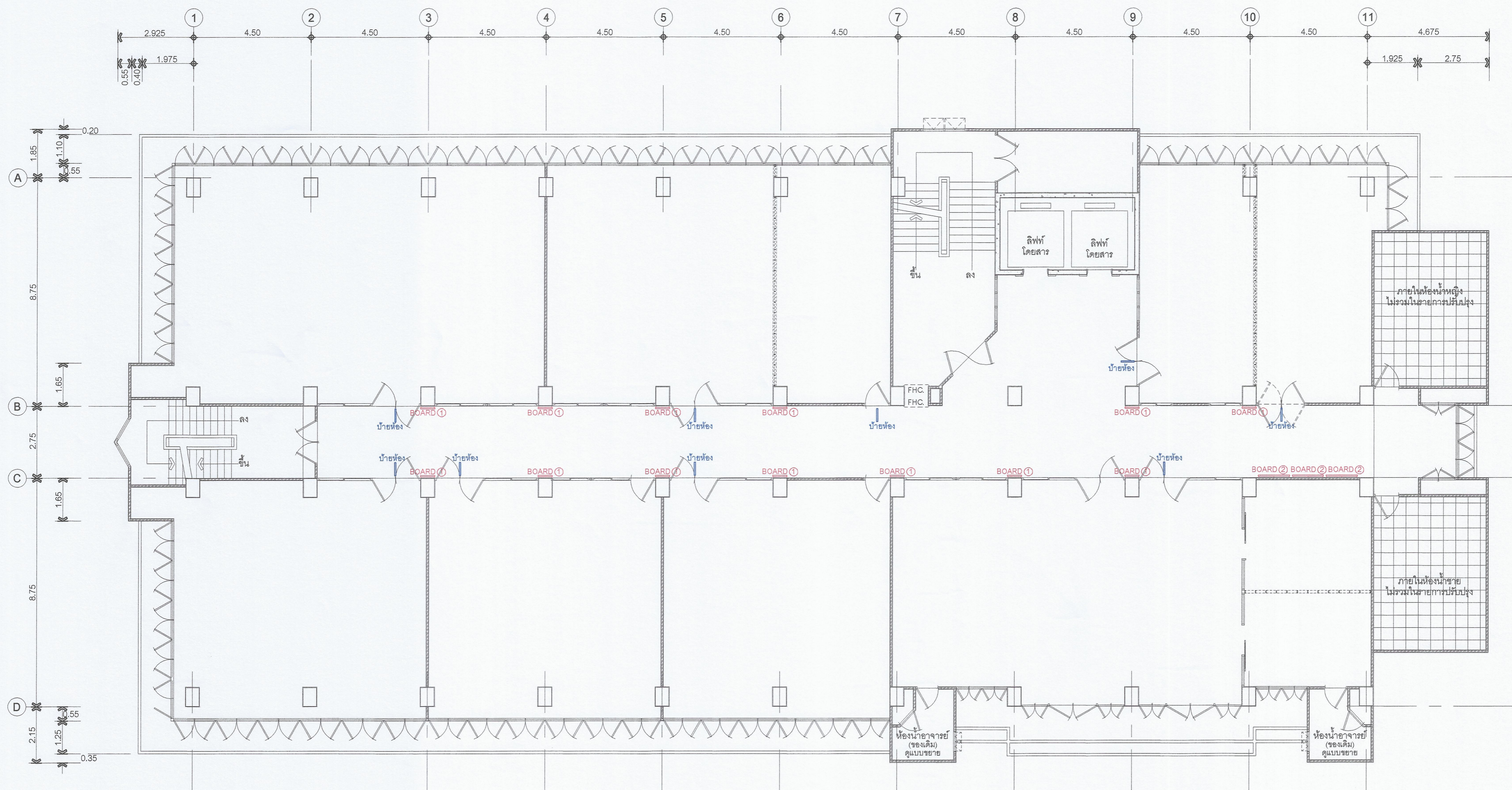
8th. FLOOR PLAN แสดงอุปกรณ์ประกอบในแต่ละชั้น หลังปรับปรุง 1 : 100
