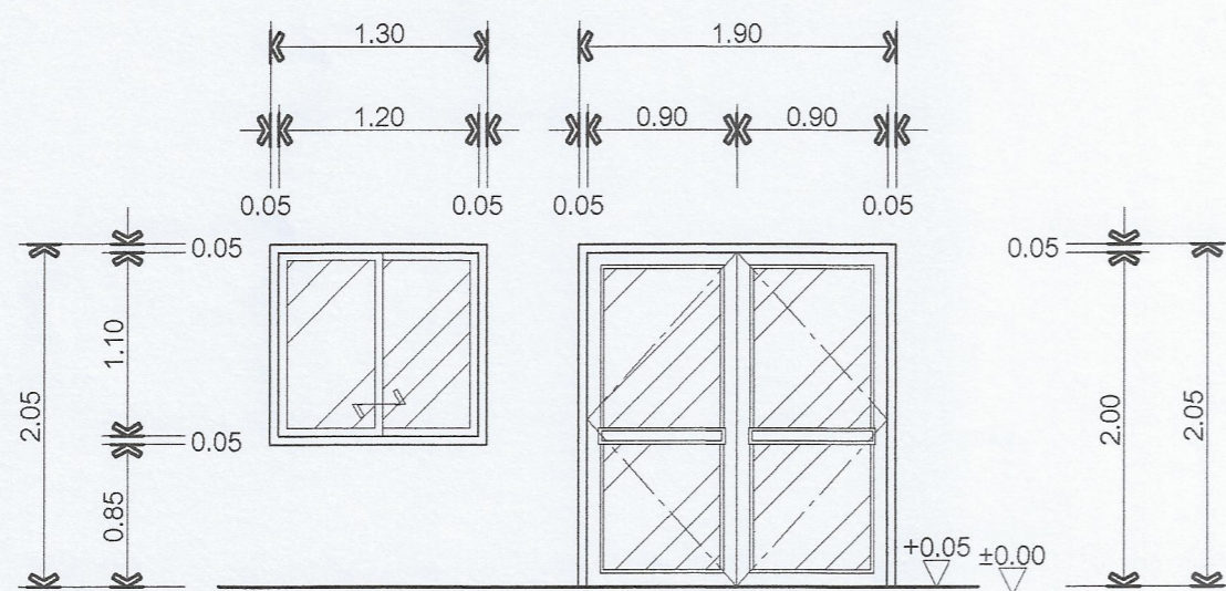
AW-ใหม่ 1:50 ห้องประชุม(801) ชั้น 8
