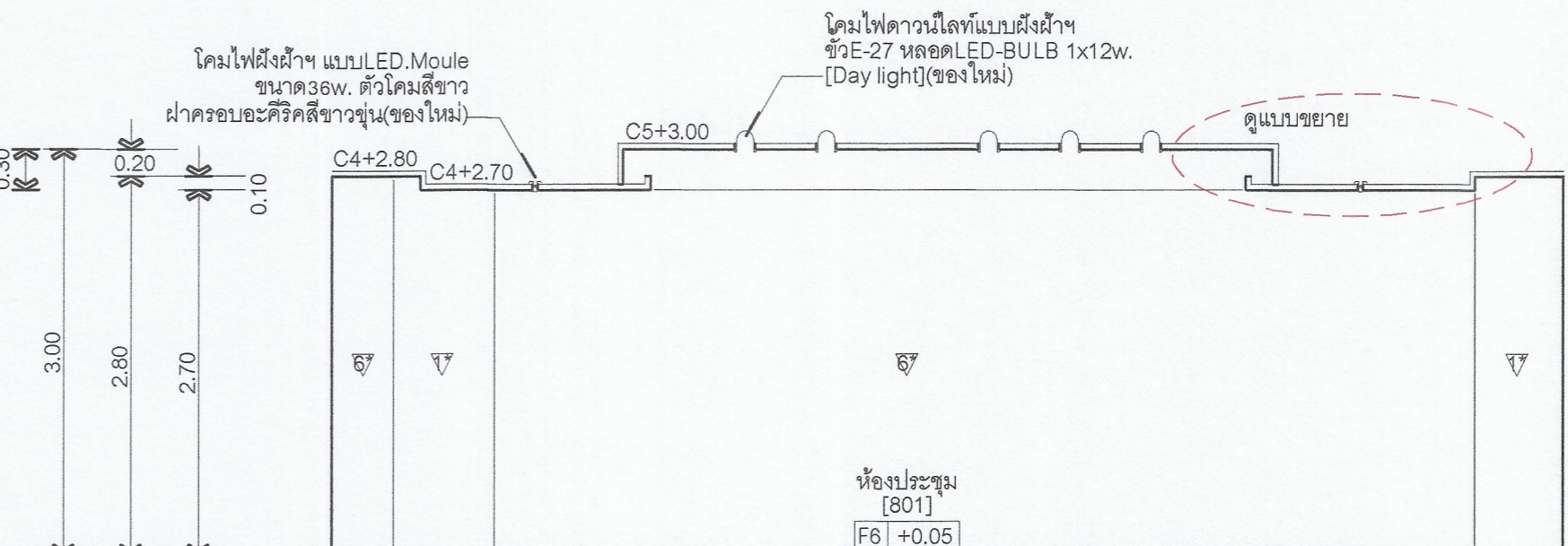
รูปด้าน [4] ห้องประชุม ชั้น 8 หลังปรับปรุง มาตราส่วน 1:50
