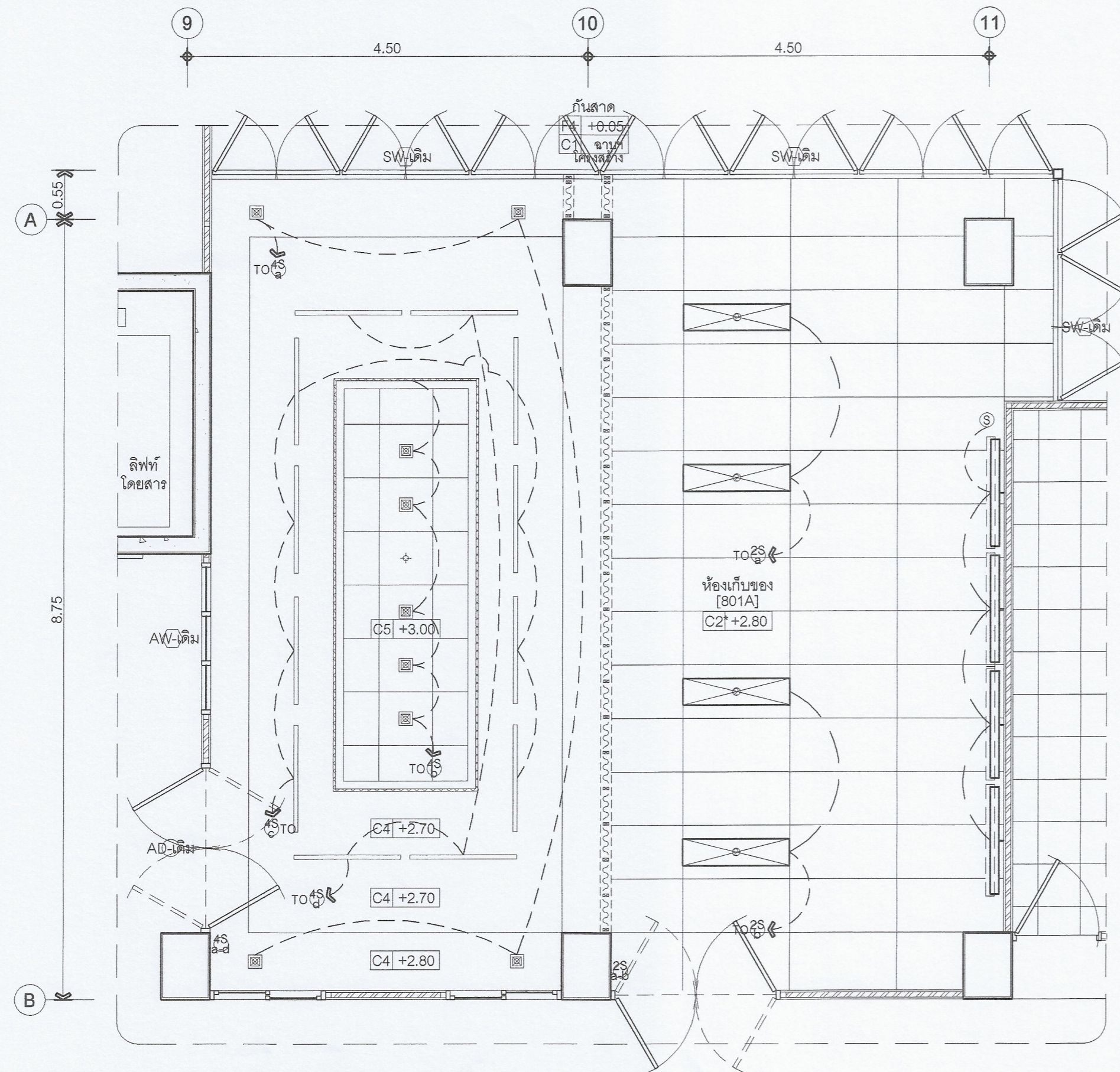
แปลนขยายห้องประชุม ชั้น 8 หลังปรับปรุง แสดงแบบโชนไฟฟ้า 1 : 50
