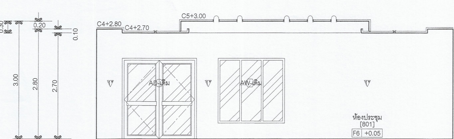
รูปด้าน [2] ห้องประชุม ชั้น 8 หลังปรับปรุง มาตราส่วน 1:50
