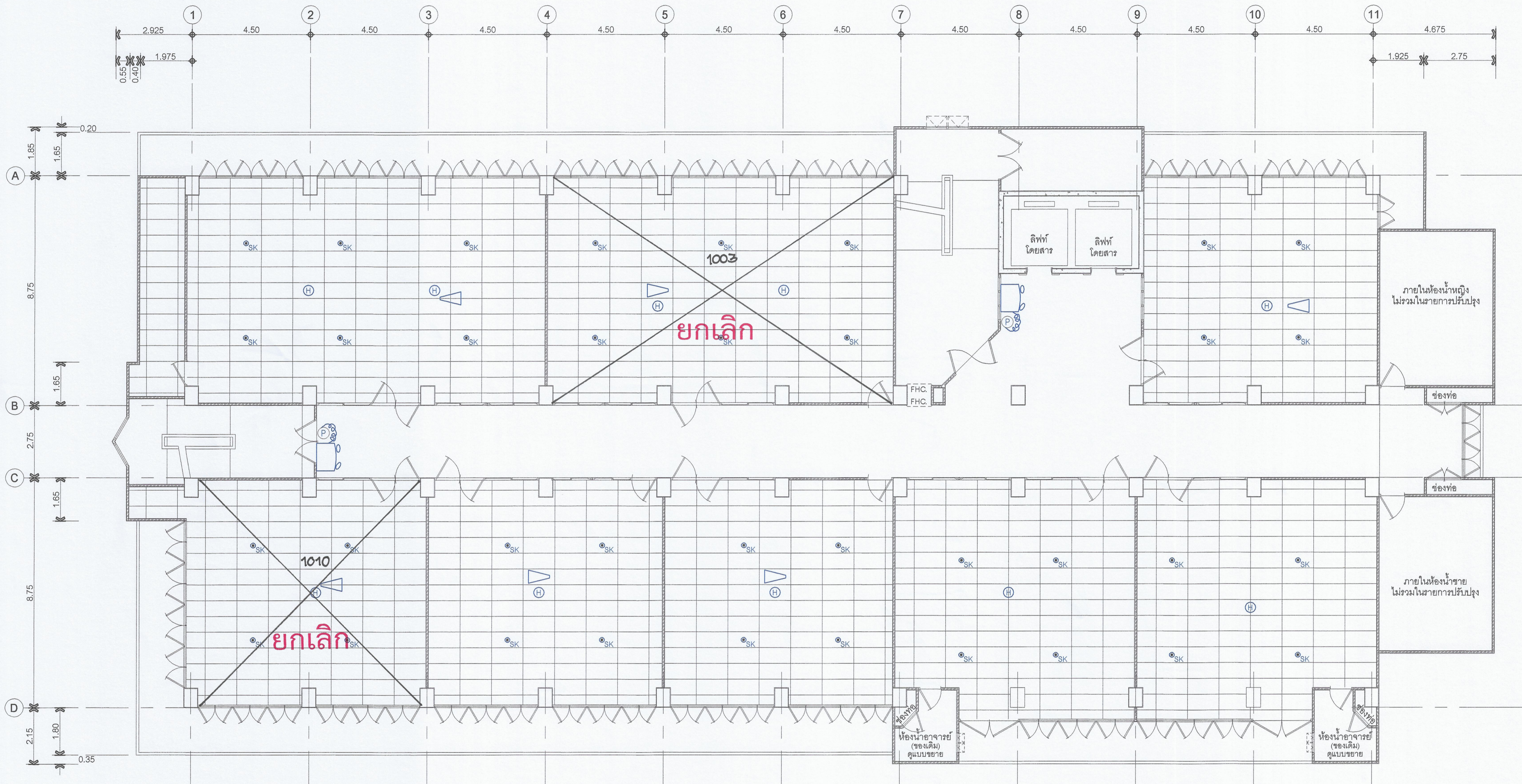
10th. FLOOR PLAN ไฟฉุกเฉิน, เครื่อง PROJECTOR SPRINKLER, HEAT DETECTOR หลังปรับปรุง มาตราส่วน 1 : 100
