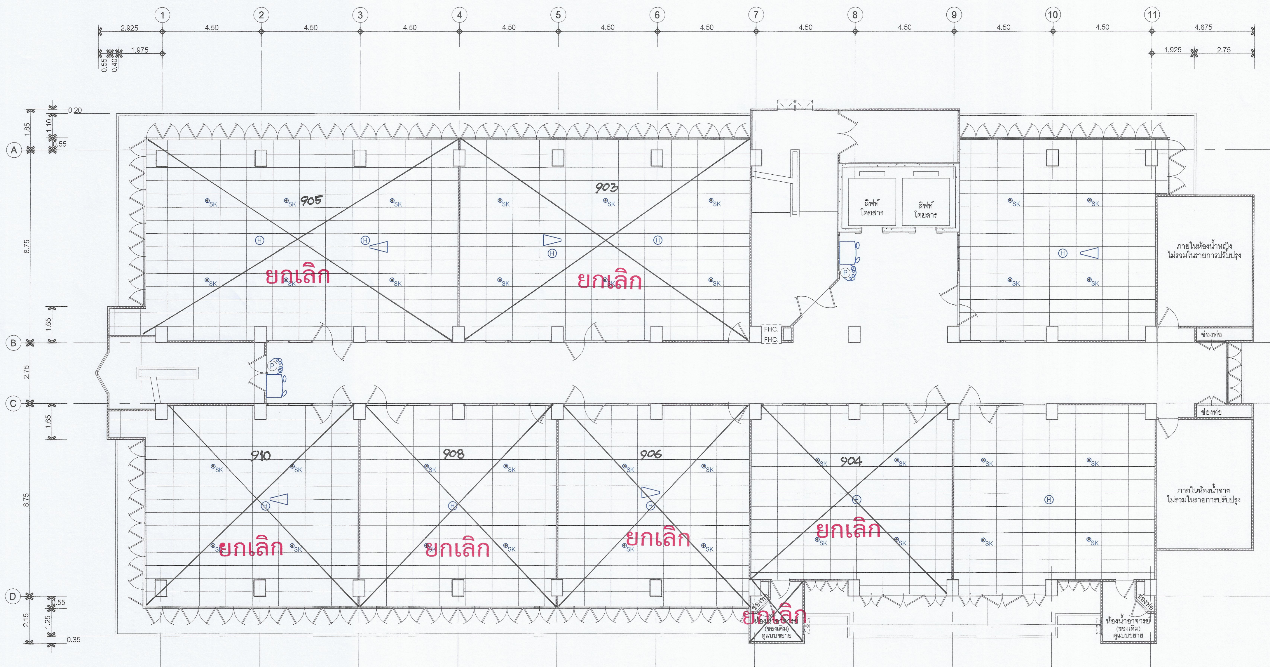
9th. FLOOR PLAN ไฟฉุกเฉิน, เครื่อง PROJECTOR SPRINKLER, HEAT DETECTOR หลังปรับปรุง มาตราส่วน 1 : 100
