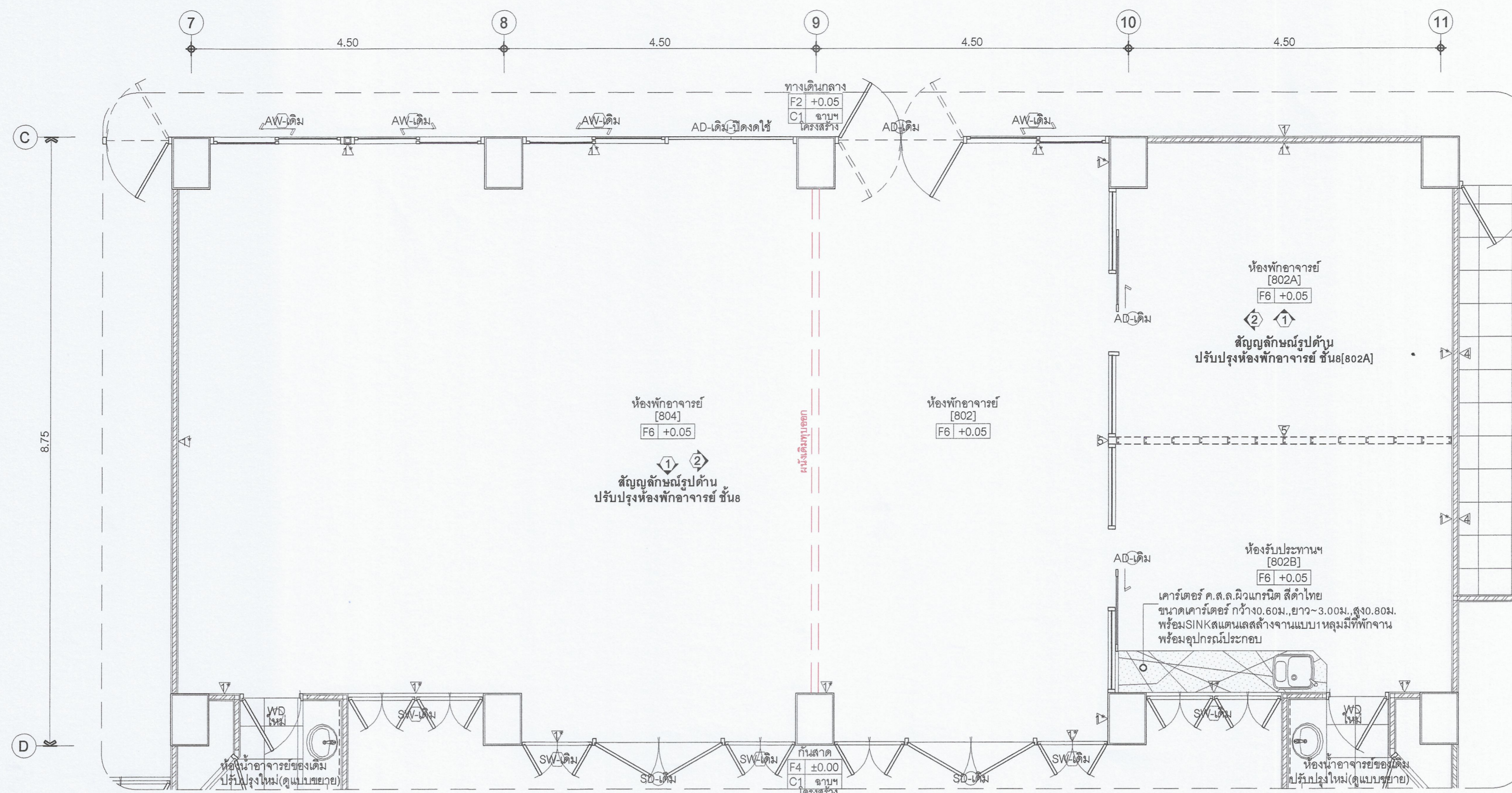
แปลนขยายห้องพักอาจารย์ ชั้น8 หลังปรับปรุง แสดงแนบโครงการ 1:50
